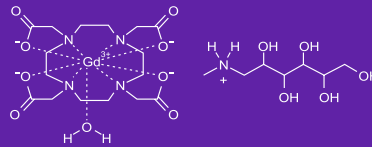
Gadoterate meglumine
